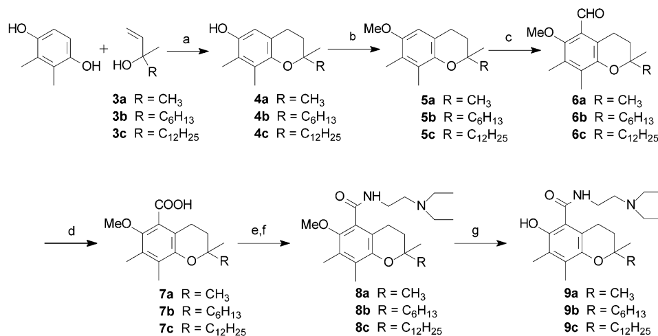
Scheme 2. (a) HCOOH, THF; (b) (MeO) 2 SO 2 , K 2 CO 3 , acetone; (c) Cl 2 CHOCH 3 , TiCl 4 , CH 2 Cl 2 ; (d) NaClO 2 , NaH 2 PO 4 ·H 2 O, H 2 O 2 ; (e) SOCl 2 , benzene; (f) N,N -diethyl-ethylenediamine, THF; (g) EtSNa, DMF.
